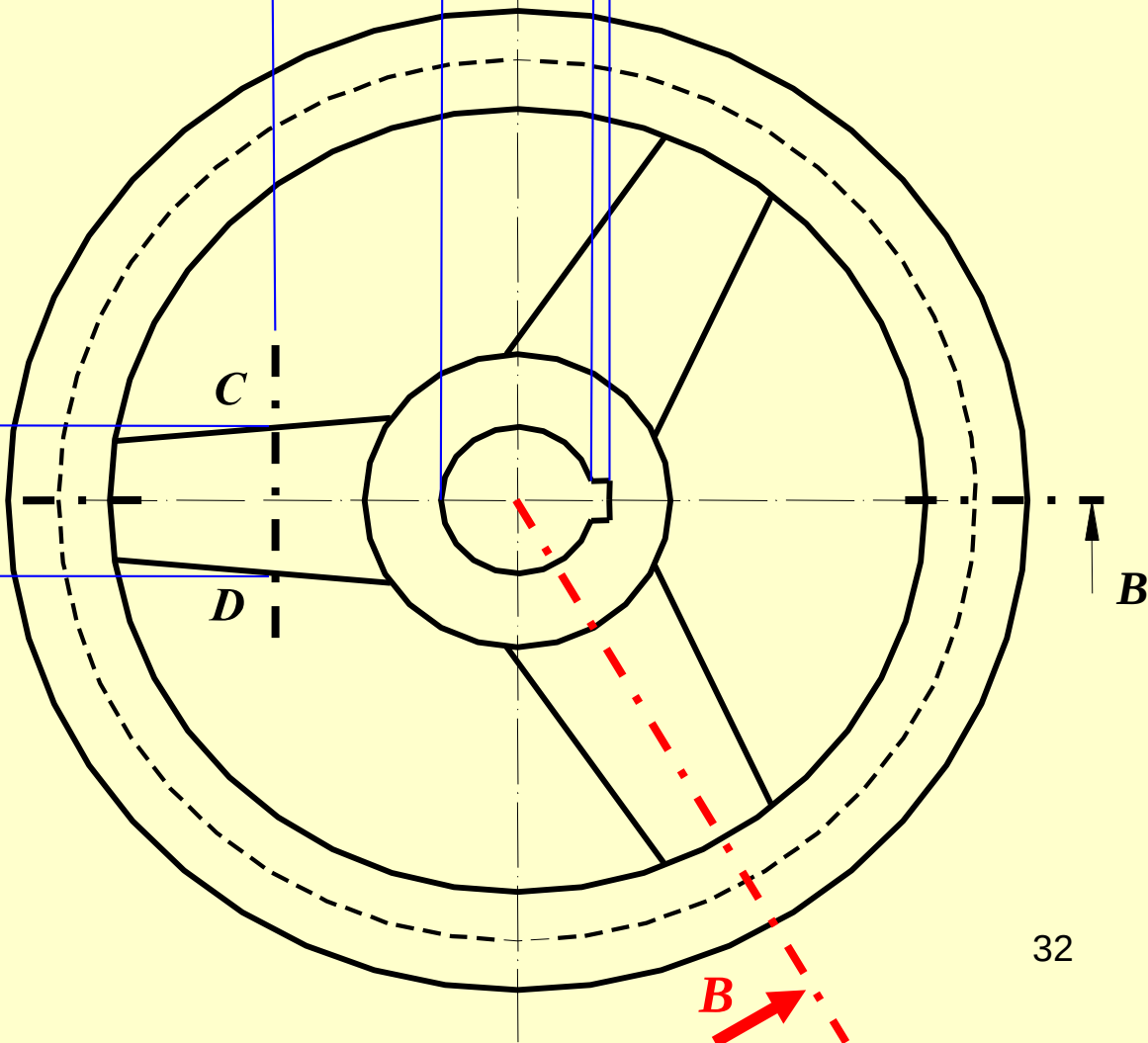
Corte - AB
