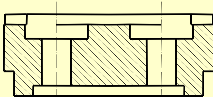
Corte - AB
