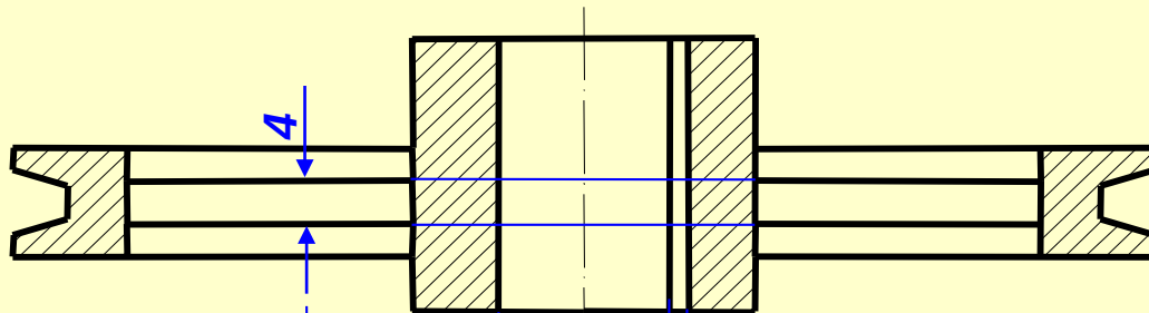
Corte - AB
